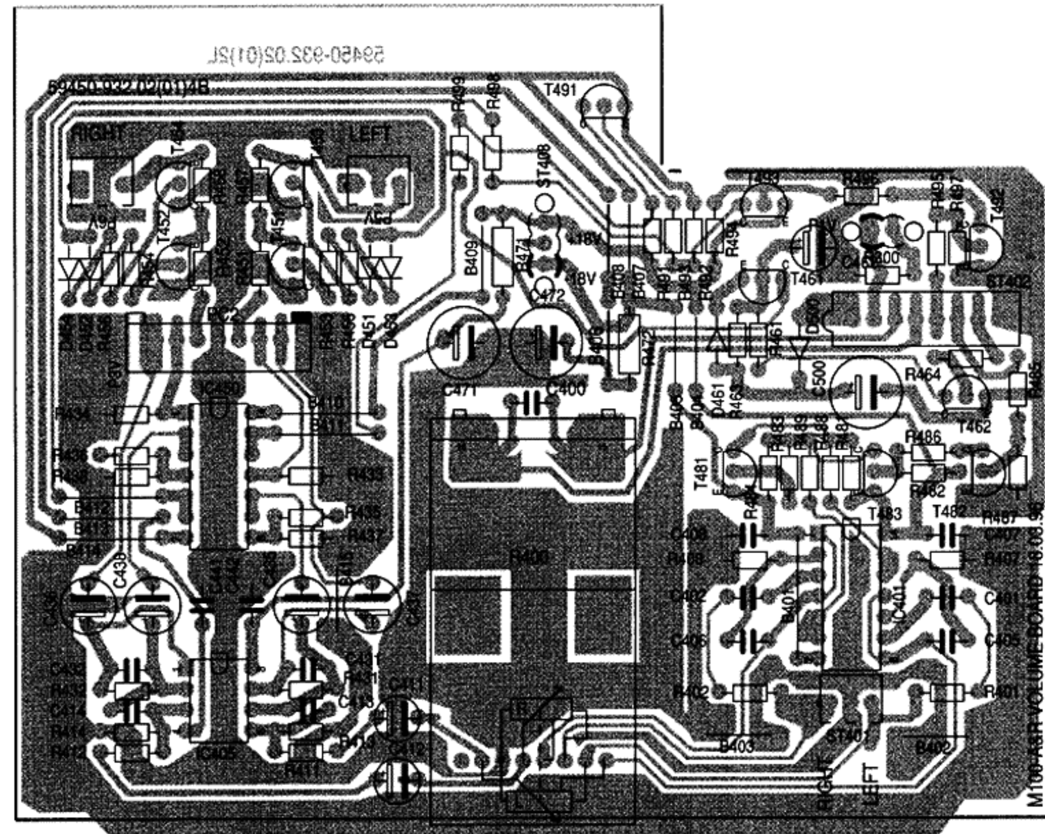
Lautstärkereglerplatte / Volume Control Board
