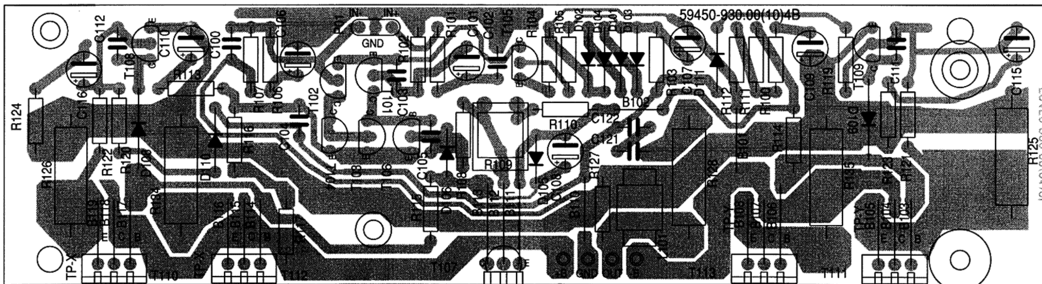
Verstärkerplatte / Amplifier Board
